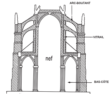
LA VOUTE GOTHIQUE
