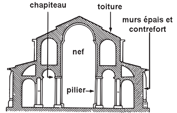
LA VOUTE ROMANE
